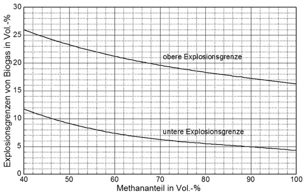
Abbildung 2: Explosionsgrenzen von Biogas in Abhängigkeit vom Methananteil /16/
