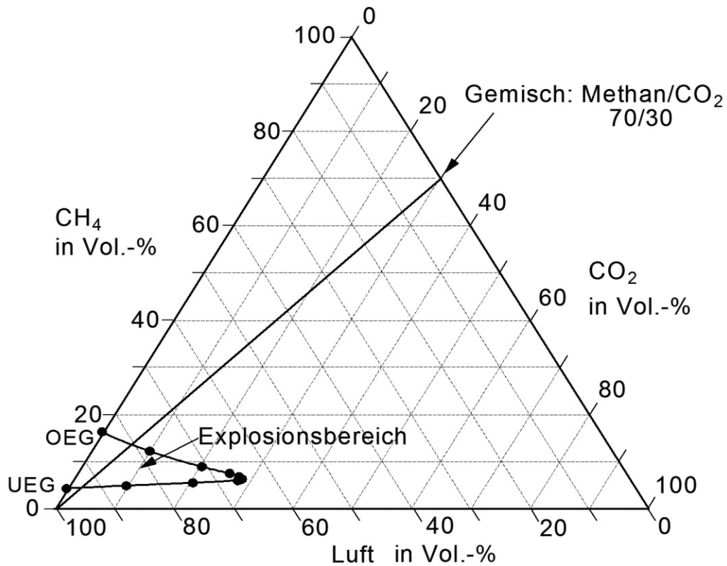
Abbildung 1: Explosionsbereich von Methan-Kohlenstoffdioxid-Gemischen – Dreiecksdiagramm /16/
